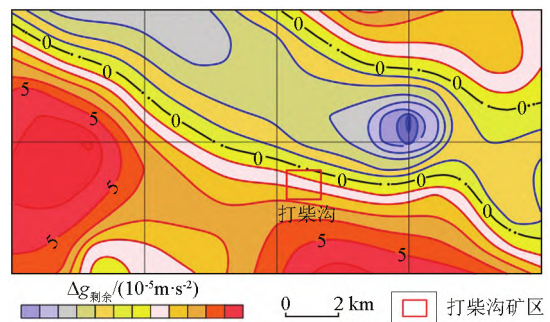
图 2 打柴沟区域剩余重力异常
