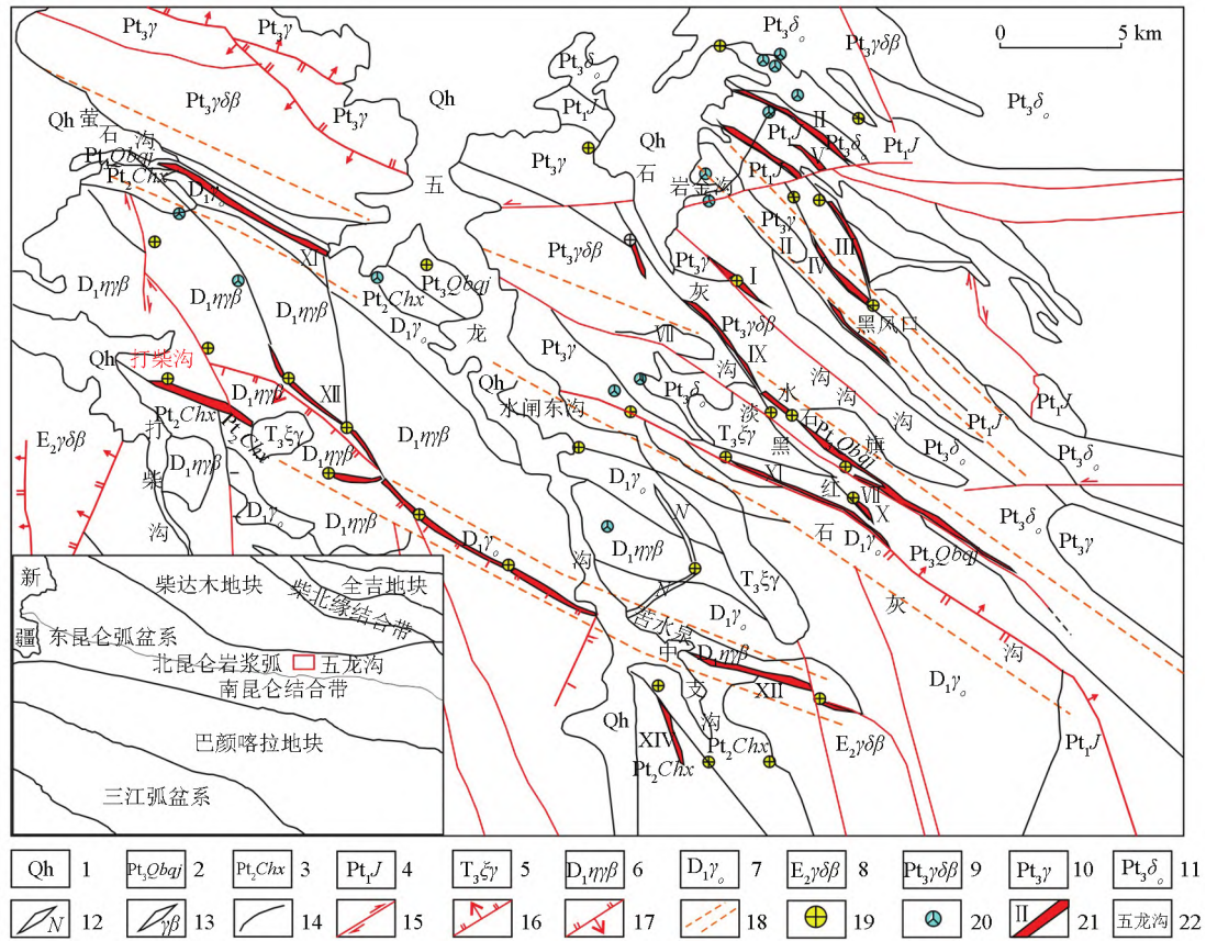
1—第四纪冲洪积物; 2—新元古代丘吉东沟组; 3—中元古代长城纪小庙组; 4—古元古代金水口岩群; 5—晚三叠世钾长花岗岩; 6—早华力西期黑云母二长花岗岩; 7—早华力西期蚀变斜长花岗岩; 8—早加里东期黑云花岗岩闪长岩; 9—新元古代黑云花岗岩闪长岩; 10—新元古代含暗色包体花岗岩; 11—新元古代石英闪长岩; 12—基性岩脉; 13—黑云母花岗岩脉; 14—地质界线; 15—走滑断层; 16—实测正断层; 17—推测逆断层; 18—韧性剪切带; 19—金矿床(点); 20—多金属矿点; 21—含金蚀变带及编号; 22—矿区位置
