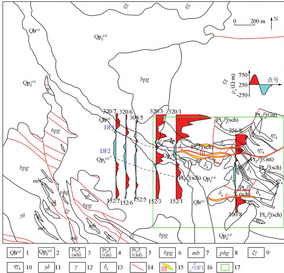
1—全新统洪冲积; 2—更新统洪冲积; 3—金水口岩群绢云石英片岩; 4—金水口岩群灰岩; 5—金水口岩群片岩夹变砂岩夹片麻岩; 6—金水口岩群灰黑色黑云斜长片麻岩; 7—金水口岩群大理岩; 8—金水口岩群灰黑色斜长角闪片麻岩; 9—正长花岗岩; 10—二长花岗岩; 11—花岗闪长岩; 12—花岗岩; 13—闪长岩; 14—断裂; 15—矿带及编号; 16—推断构造; 17—打柴沟矿区
