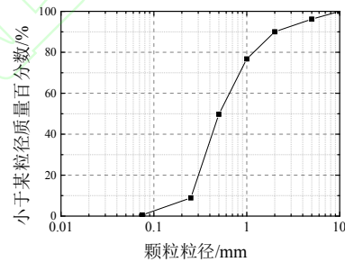
图 3 砂土粒径级配曲线
