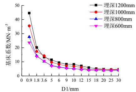
图 15 辅助观测面内土体水平基床系数
