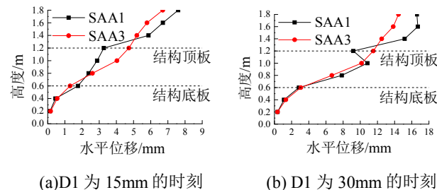
图 11 SAA 上不同高度测点的水平位移
