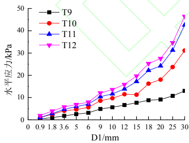
图 13 辅助观测面内土体水平应力
