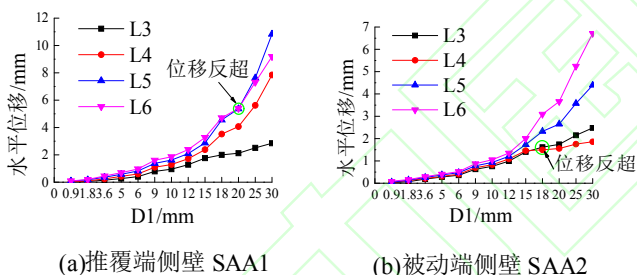
图 9 结构侧壁水平位移
