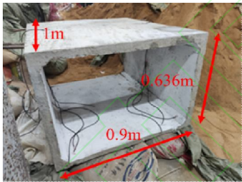
图2 试验模型实物图
