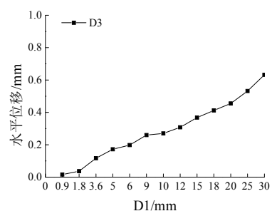
图 5 被动端滑板水平位移
