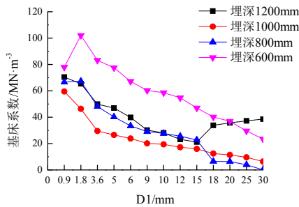
图 16 推覆端侧壁水平基床系数
