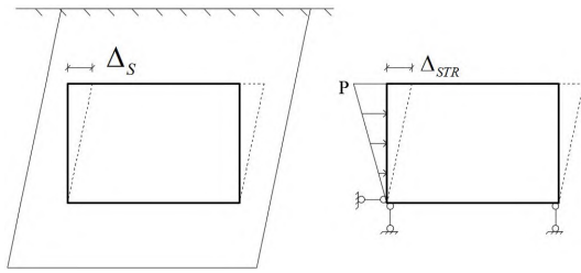
图 12 相互作用系数法计算模型
