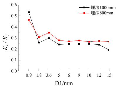
图 17 土体与结构水平基床系数比值
