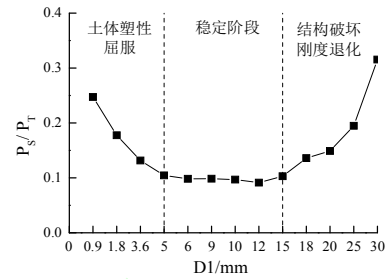
图 14 土体荷载与结构荷载比值
