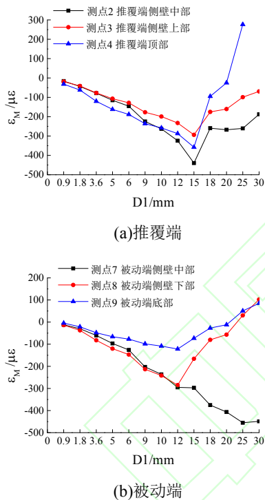
图 6 模型结构应变响应
