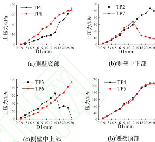
图 10 结构侧壁水平土压力
